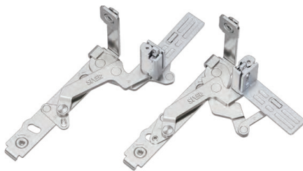
נבדק ב-250,000 מחזורי פתיחה
